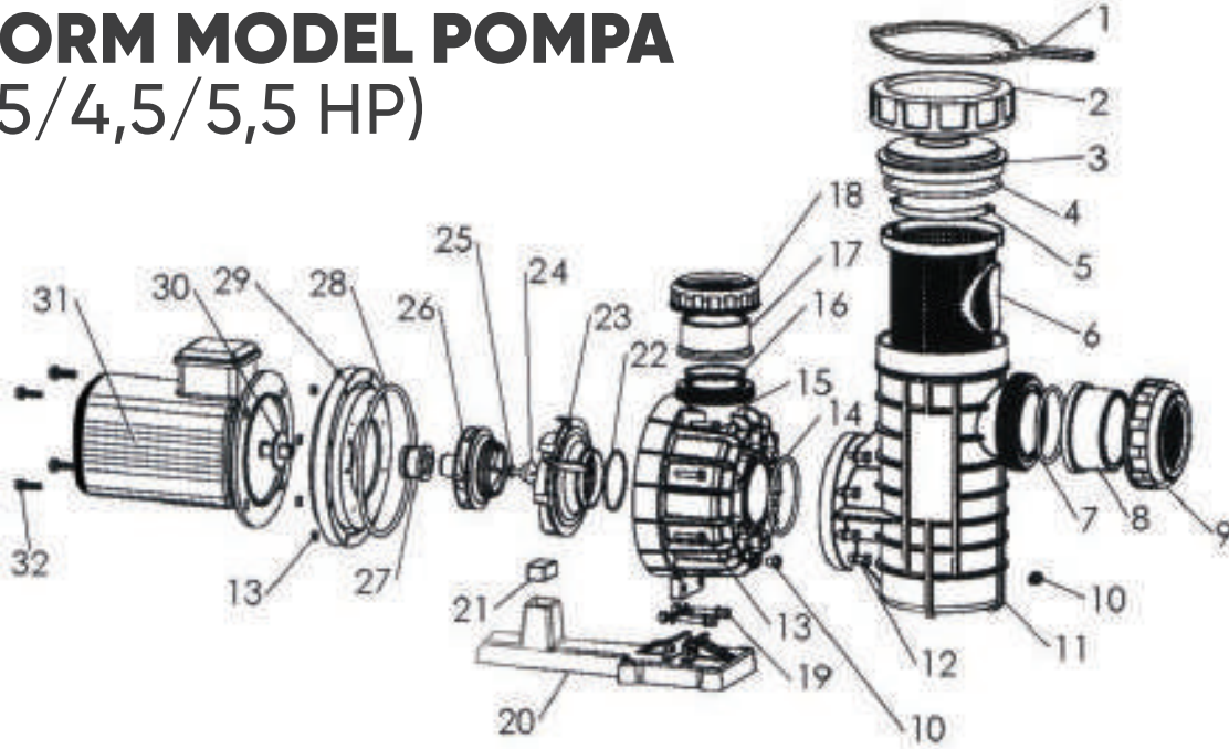
Atlaspool Havuz Pompaları Yedek Parça Listesi
