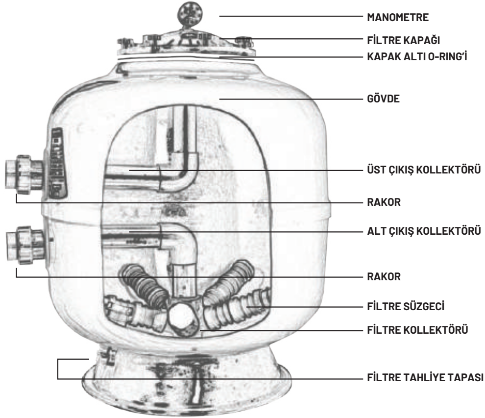
Atlaspool Havuz Filtreleri Yedek Parça Listesi
