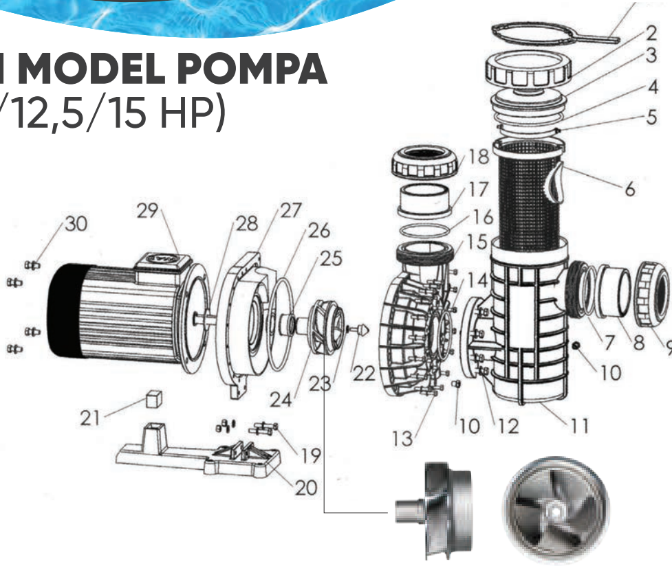
Atlaspool Havuz Pompaları Yedek Parça Listesi
